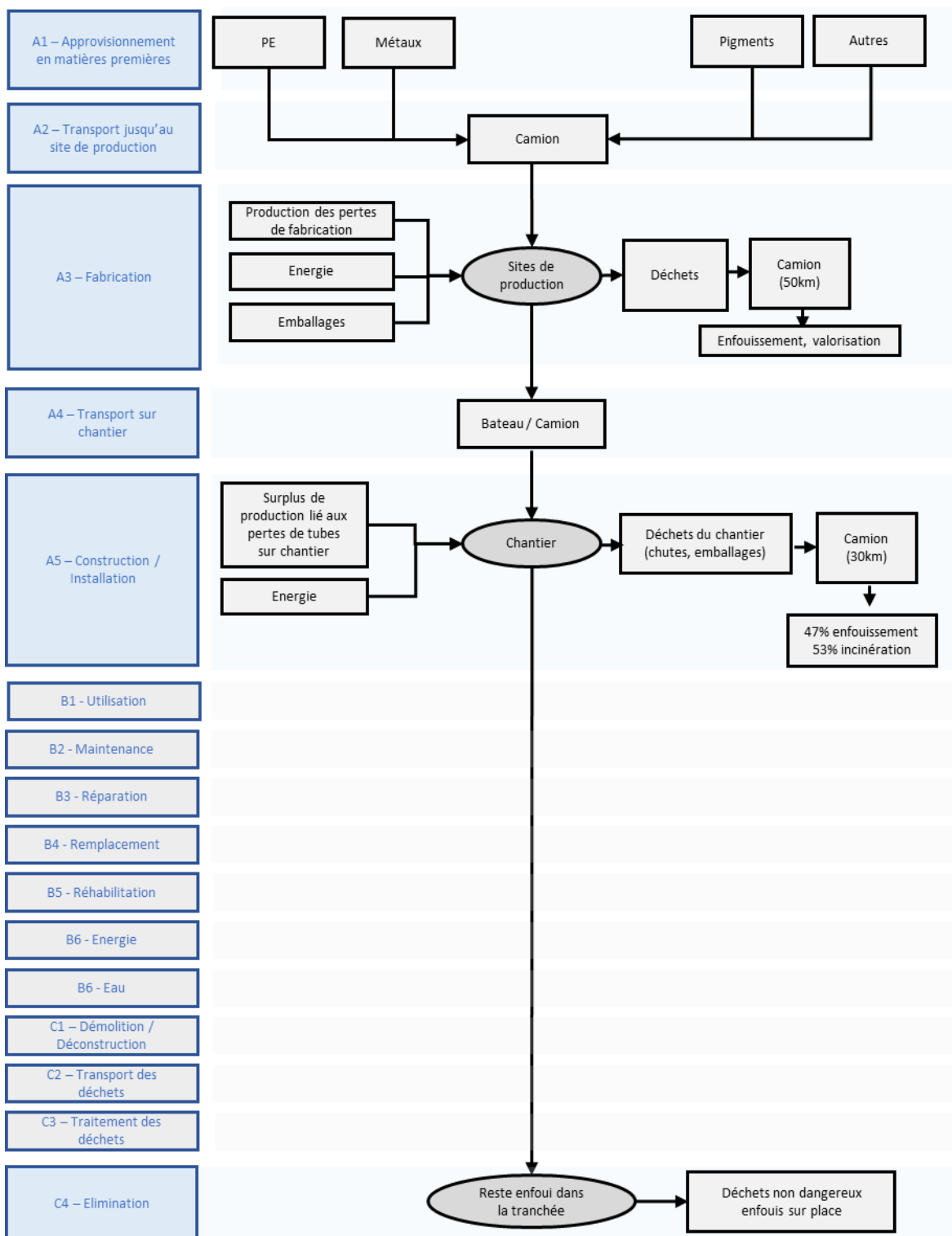
Figure 1 – Diagramme simplifié du cycle de vie du produit
